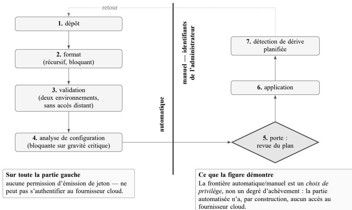
FIG. 4. Chaîne de provisionnement de l’infrastructure : la frontière automatique/manuel comme choix de privilège
